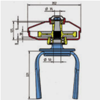
Schräges Wannenprofil der Zirkon 8
