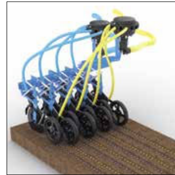
Abb. 2: Zwei Komponenten werden jeweils über ein eigenes Säschar ausgebracht
