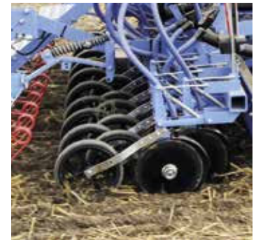
Doppelscheibenschar
