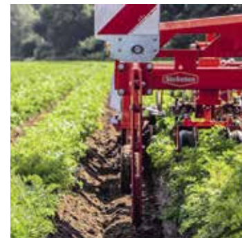
Optionaler Tiefenlockerer zur Lockerung des Bodens zwischen den Dämmen
