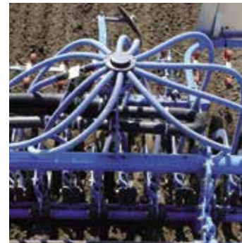
Saatgutverteiler
